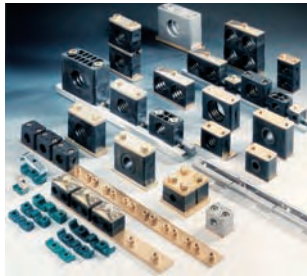
Befestigungsschelle DIN 3015 Mounting clamps DIN 3015 Colliers DIN 3015
